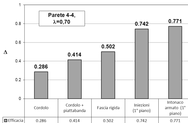
Figura 2.60 – Parete 4-4 con fascia di piano debole: incremento di resistenza atteso in funzione dei diversi interventi
