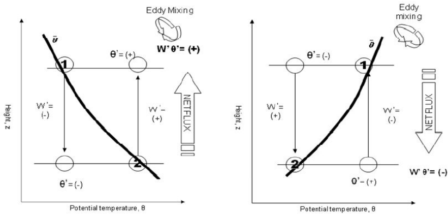
Figura 5.1-1 schema semplificato delle misure eddy covariance
