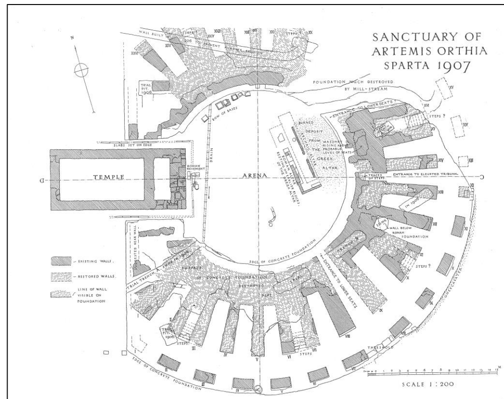
Pianta eseguita al termine della seconda campagna di scavo Da DAWKINS 1906-1907, Tav. II
