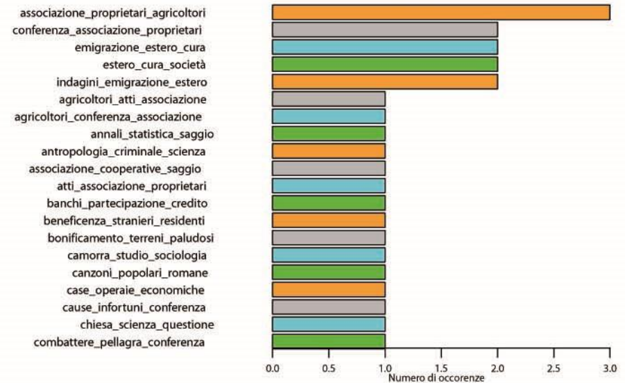
Inchieste Sociali 1890 – Trigrams (funzioni base)
