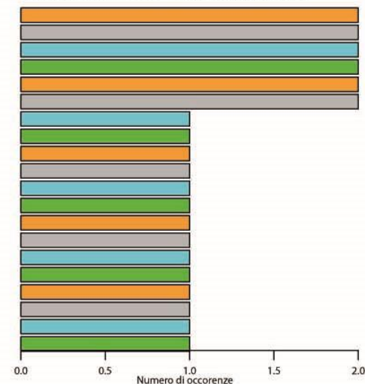
Inchieste Sociali 1913 – Trigrams (funzioni base)
