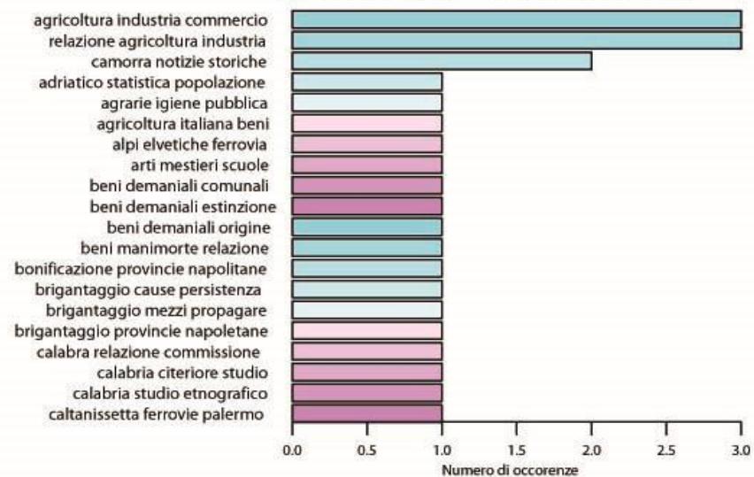
Inchieste Sociali 1862 – Trigrams (funzioni base)
