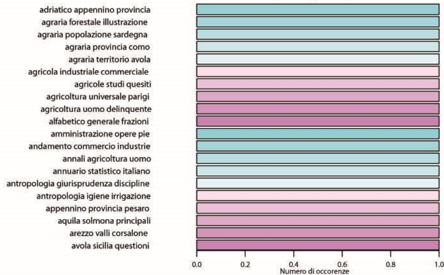
Inchieste Sociali 1878 – Trigrams (funzioni base)
