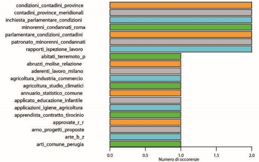
Inchieste Sociali 1909 – Trigrams (funzioni base)
